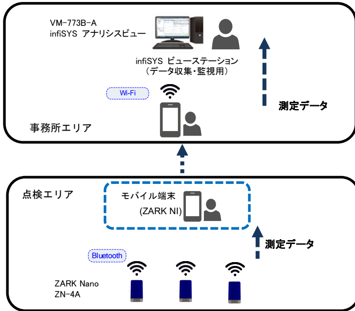
図 1 システム構成例
