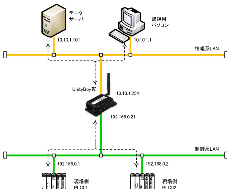
図1.2-1 増設LAN I/Fカードを用いたネットワーク構成イメージ
