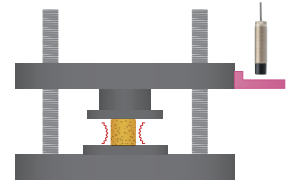
圧縮試験機、 引張試験機の変位計測
