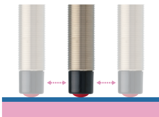
塗膜厚さ計測、 シート・フィルム厚さ計測
