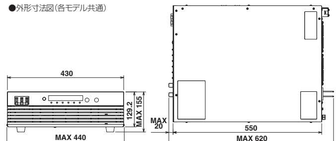
●外形寸法図 (各モデル共通)
